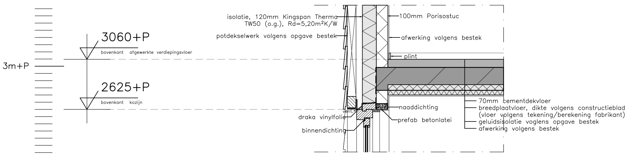
Detail kozijn/potdekselwerk
