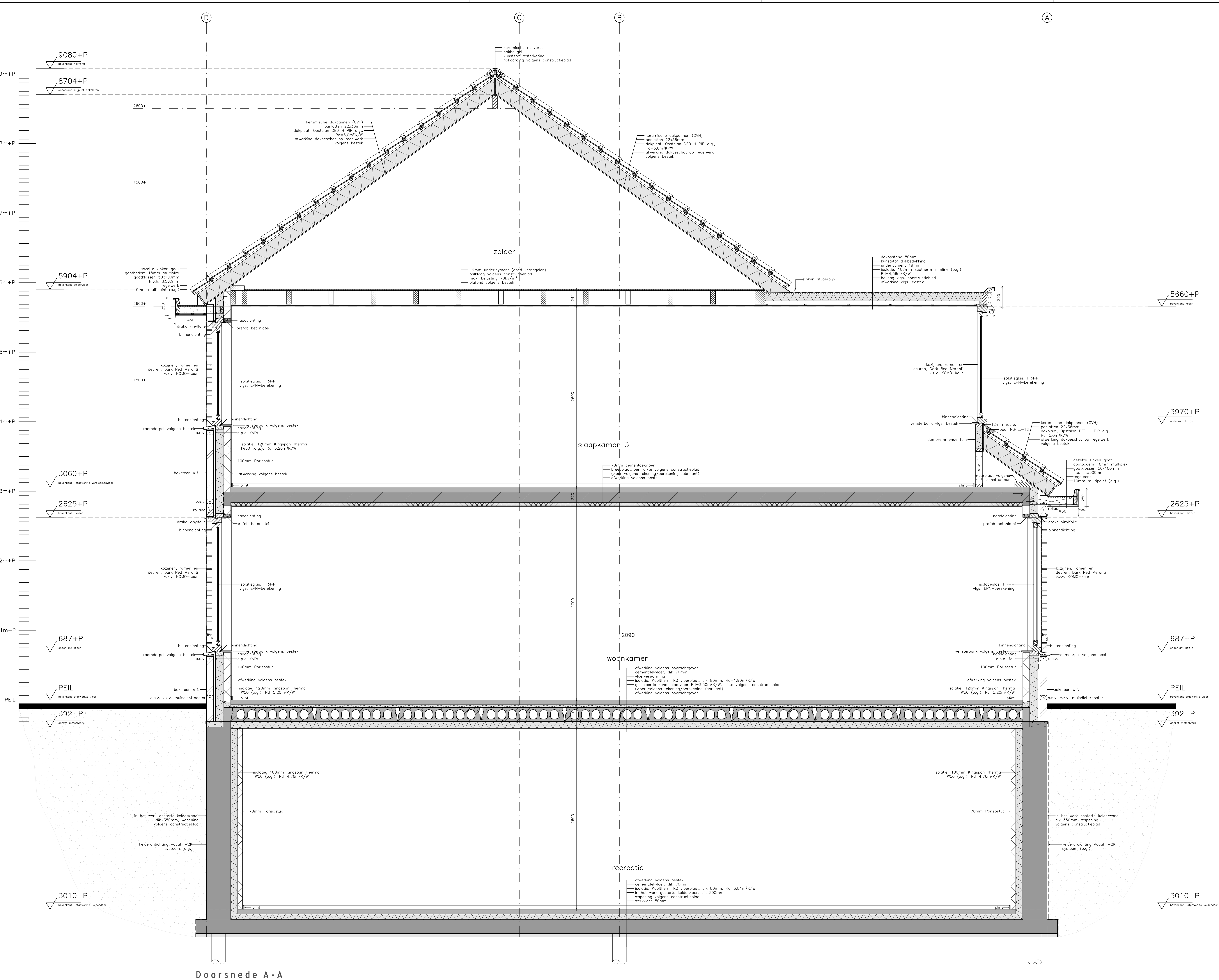
Doorsnede A-A
