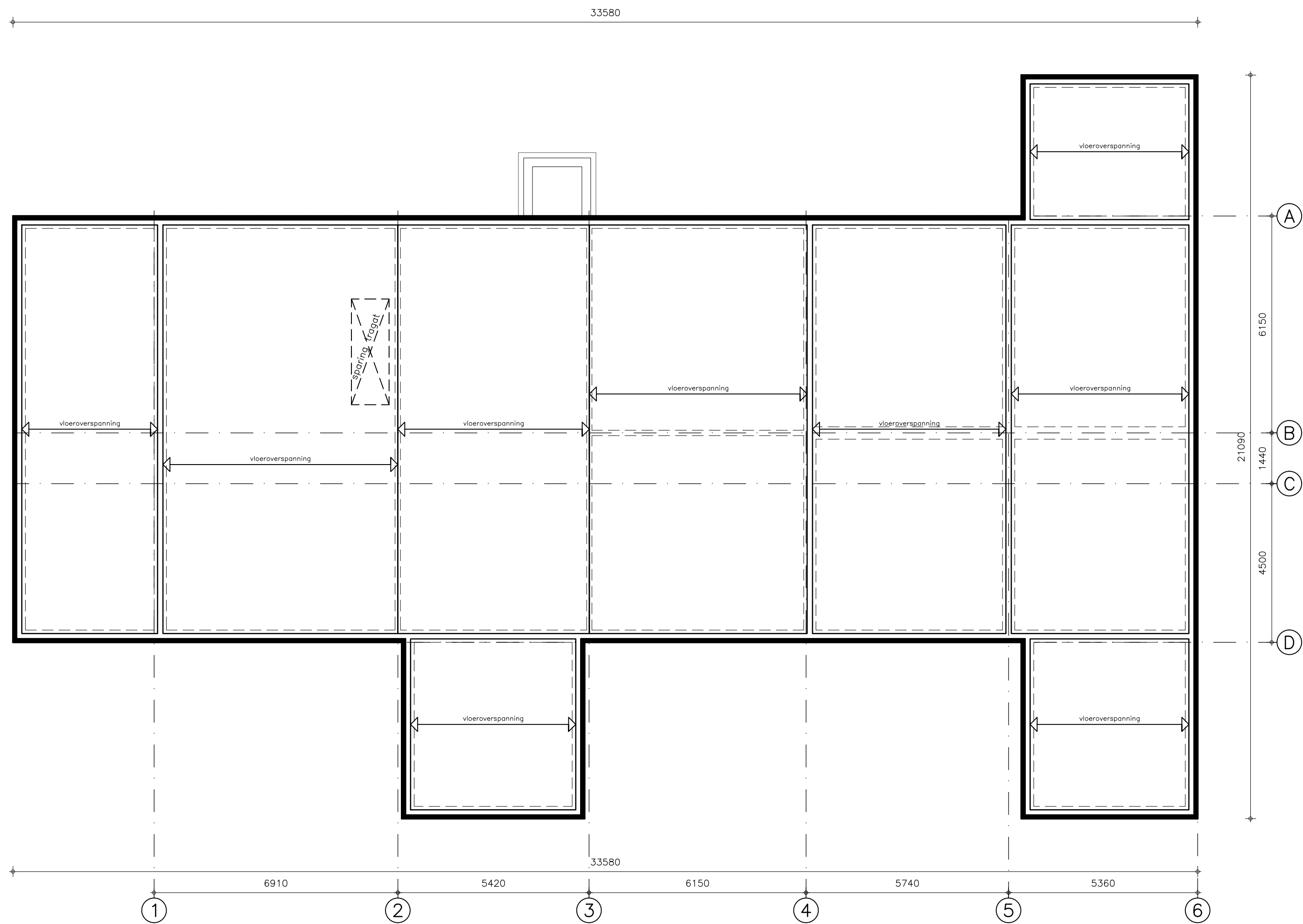
Begane grondvloer
