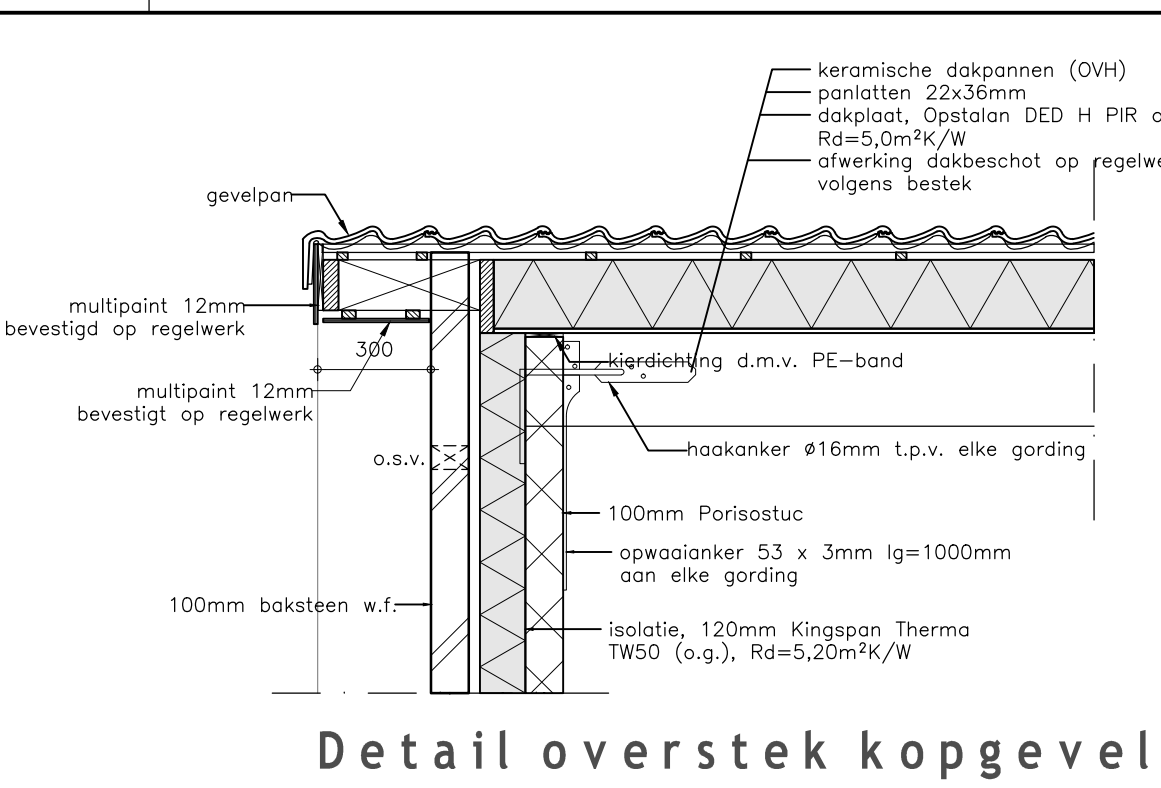
Detail overstek kopgevel
