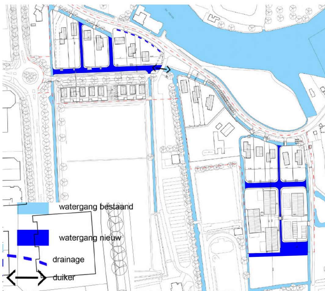
Figuur 5.1 Nieuwe waterstructuur plangebied.
