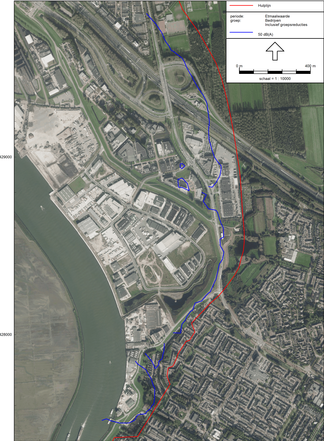
Figuur 4 50 dB(A) geluidcontour (Blauw) In relatie tot zonegrens (rood)
