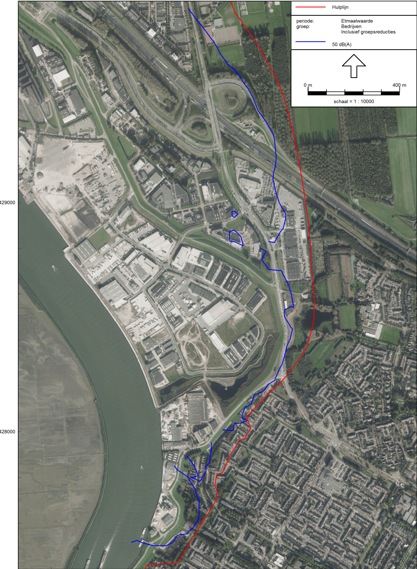
Figuur 5 50 dB(A) geluidcontour (Blauw) In relatie tot zonegrens (rood)
