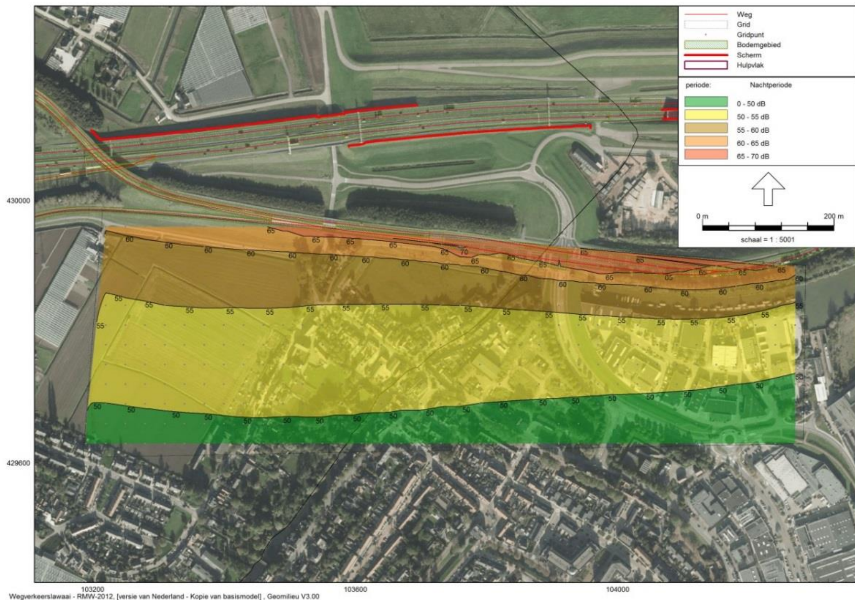
Figur 3 Geluidcontour nachtperiode
