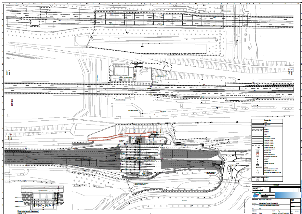
Figuur 1: Het ontwerp van het tolplein.
