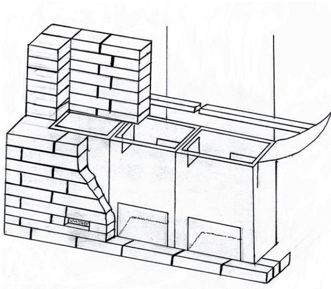
Doorsnede Ingemetselde vleermuisvoorzieningen Buitenaanzicht inpandige voorzieningen.
