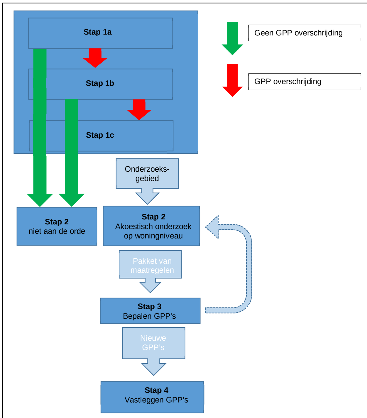
Figuur 5.1 Schematisch overzicht werkwijze bij wijziging van een weg
