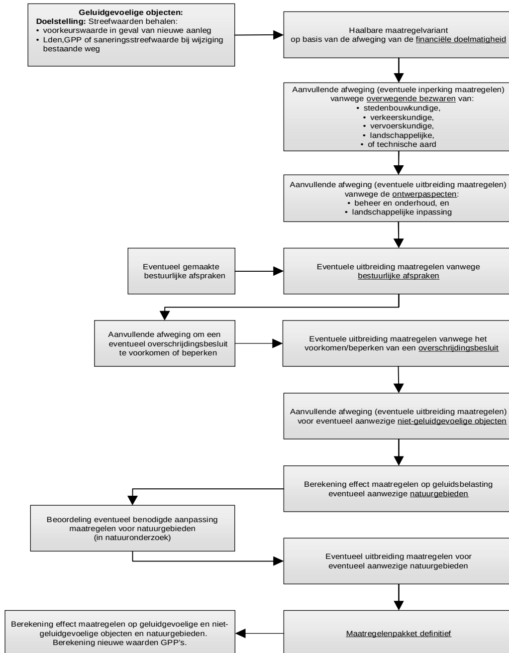
Figuur 2.1 Stroomschema van de methodiek voor het bepalen van de maatregelenvariant
