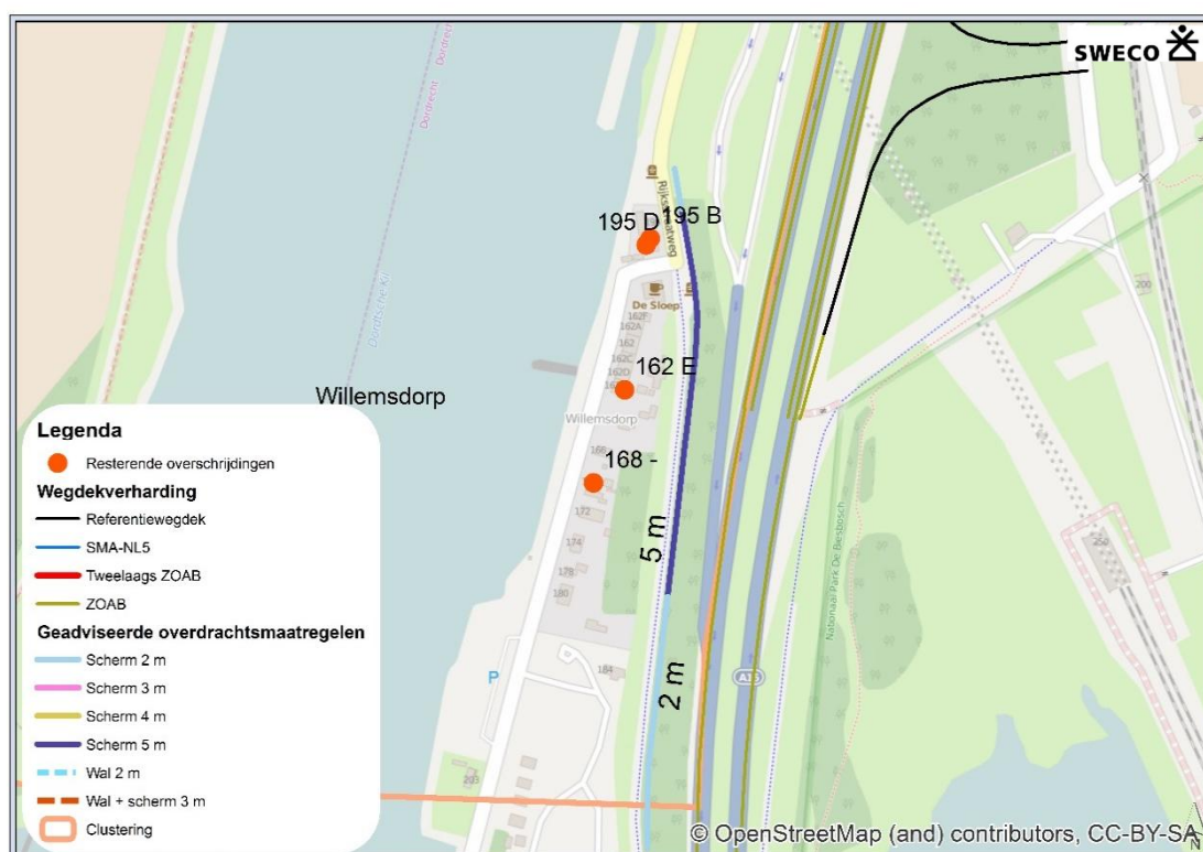
Figuur 7.16 Cluster 'Willemsdorp' na maatregelen
