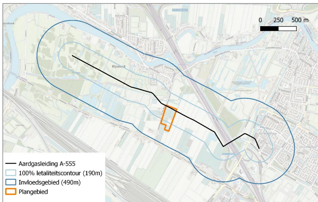
Figuur 2. Invloedsgebied en 100%-letaliteitscontour aardgasleiding A-555
