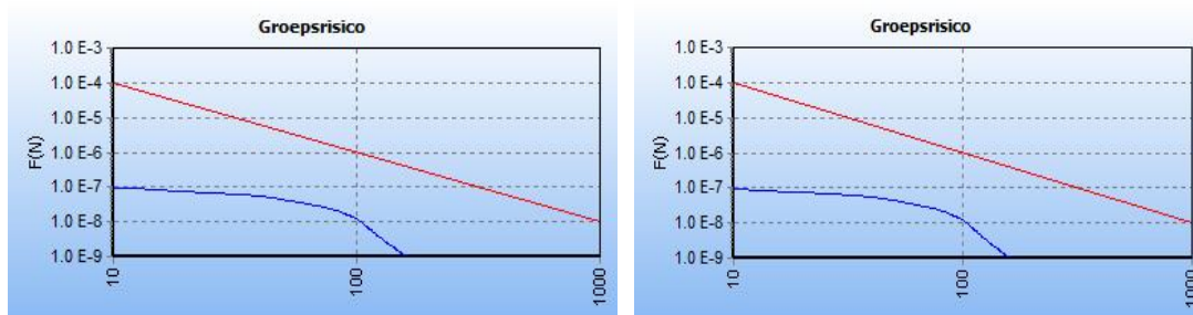
Figuur 4. Groepsrisico A-555, huidig (links) en toekomstig (rechts)
