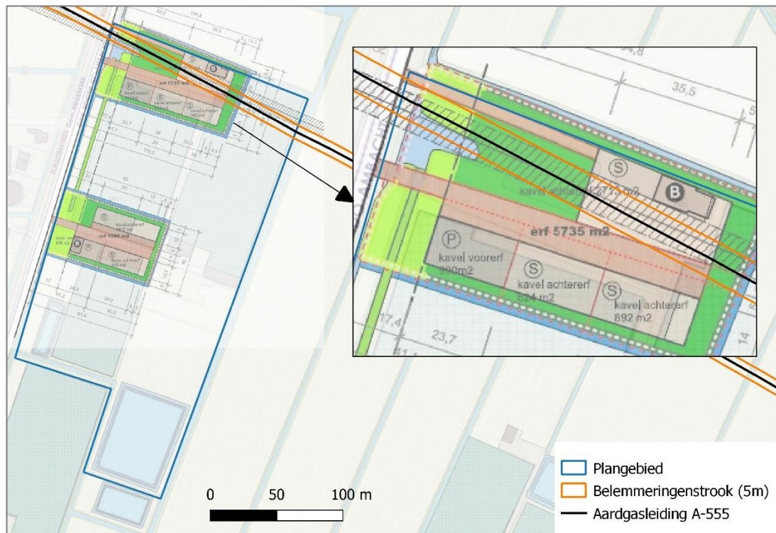
Figuur 5. Belemmeringenstrook van aardgasbuisleiding A-555
