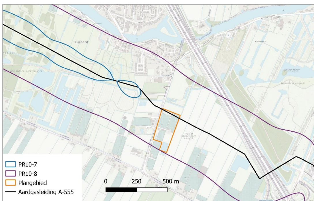
Figuur 3. Plaatsgebonden risicocontouren aardgasleiding A-555
