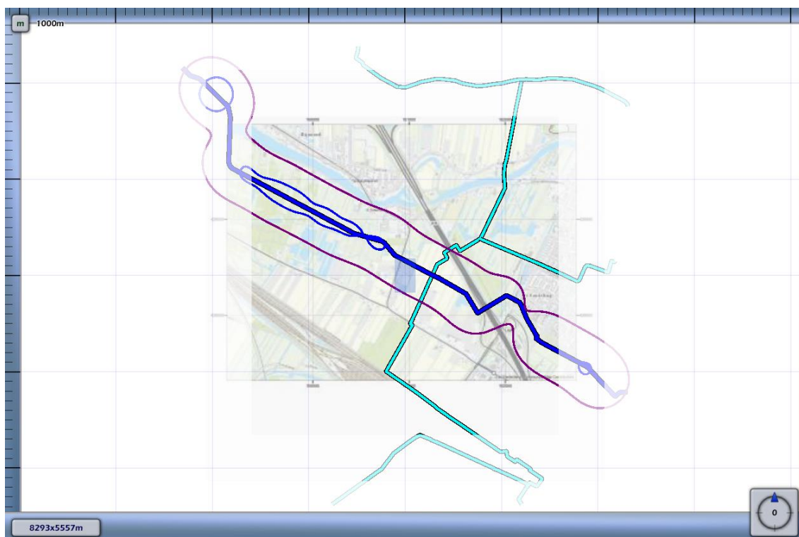
3.1 Figuur 3.1 Plaatsgebonden risico voor 6615_leiding-A-555-deel-1 van N.V. Nederlandse Gasunie
