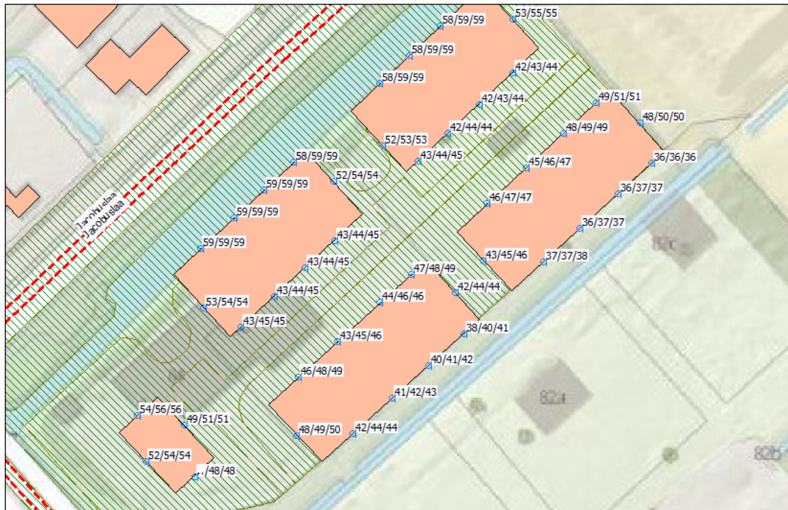
Figuur 3: Cumulatieve geluidbelasting L_{cum} van alle in het onderzoek betrokken wegen
