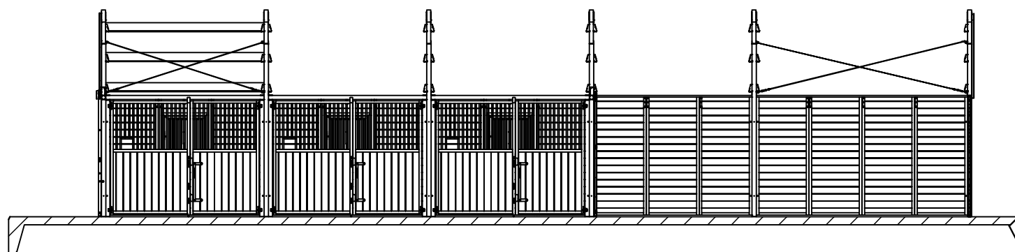
A-A ( 1 : 100 )
