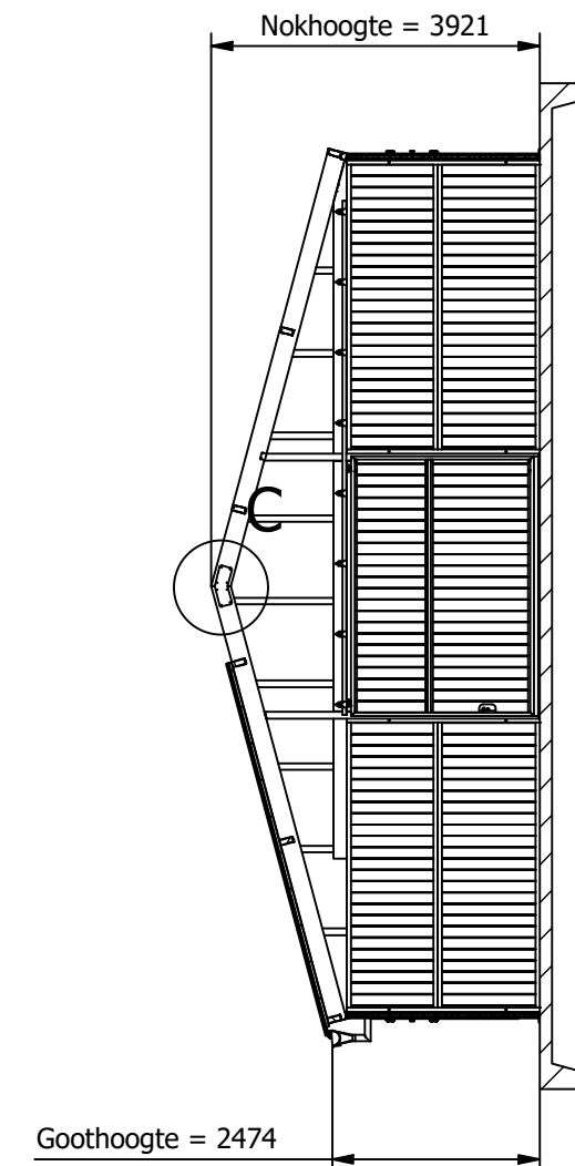
B-B ( 1 : 100 )
