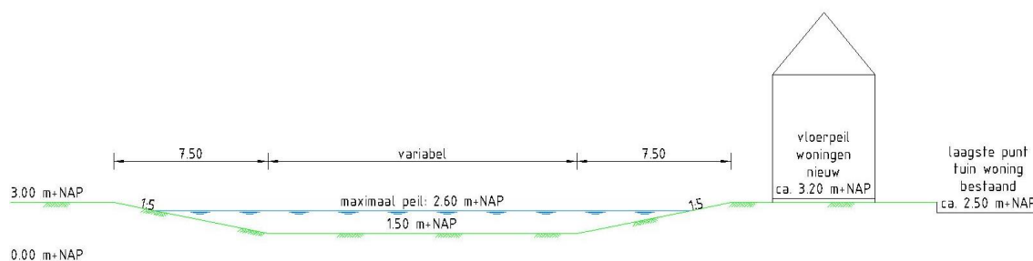
Principedoorsnede bergingsvijver woonarken
