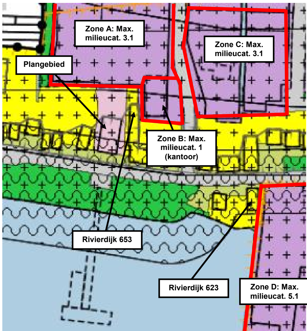
Afbeelding 16: Zoning bedrijventerrein
