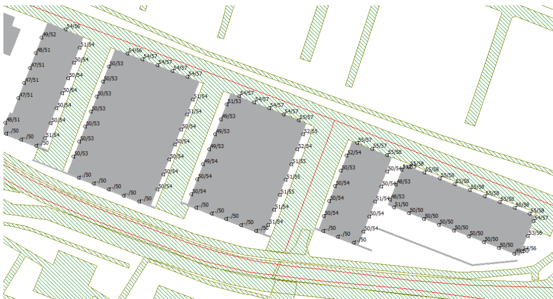
Figuur 4.1 Geluidsbelasting ten gevolge van het verkeer op de A15 exclusief correctie artikel 3.4 Rmg
