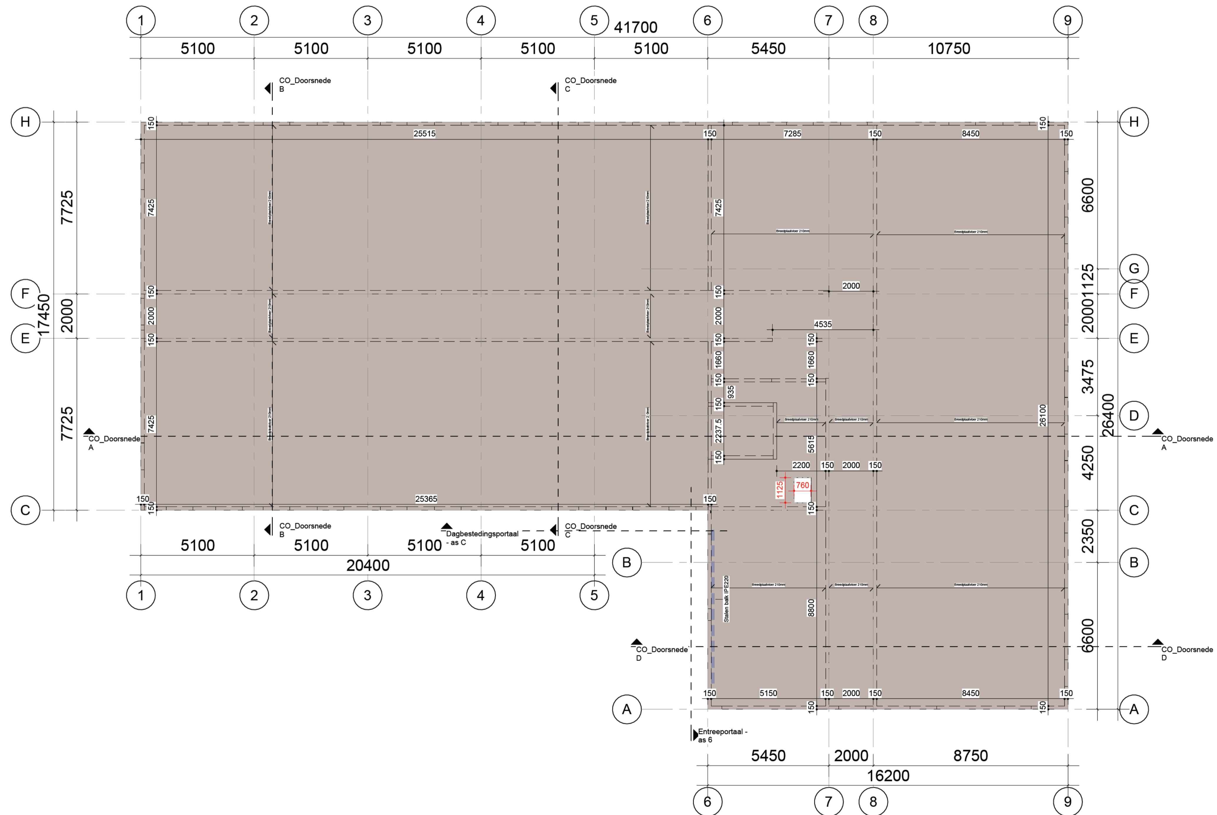
02 Dak CO schaal 1 : 100
