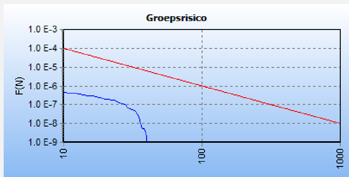
Figuur 6.3 FN curve voor buisleiding W-530-05 van Gasunie voor de kilometer tussen stationing 400.00 en 1400.00 (bestaande en nieuwe situatie)
